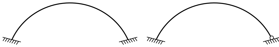
Eingespannter Bogen (stat. unbestimmt)
