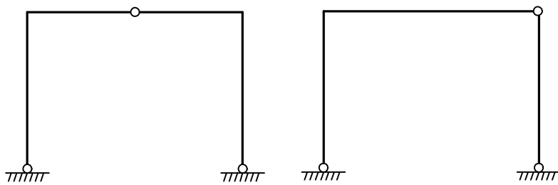
Dreigelenk Rahmen (statisch bestimmt)
