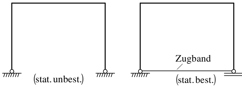
Zweigelenk Rahmen (mit oder ohne)
