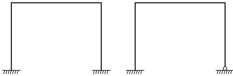
Eingespannter Rahmen (statisch unbestimmt)
