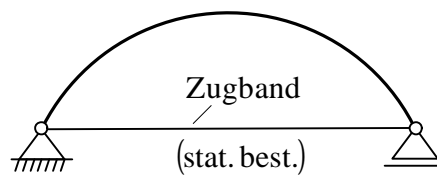
Zweigelenbogen (mit und ohne Zugband)
